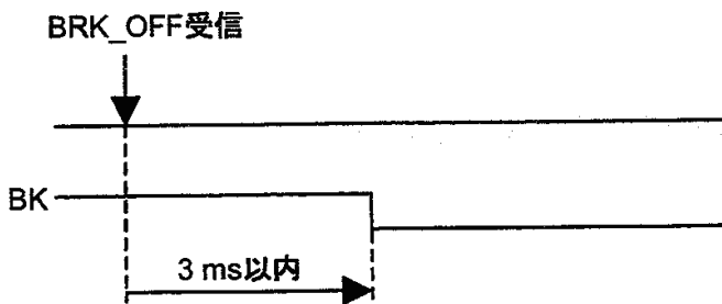
制动解除信号的时序
